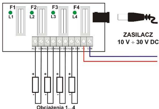
Rys.1. Schemat podłączenia modułu (przykładowy).
