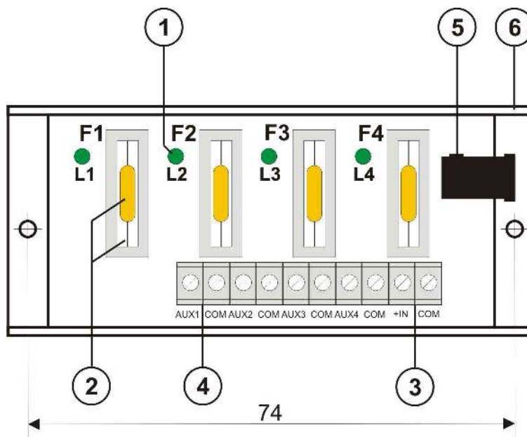
Rys.2. Widok modułu.
